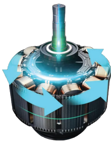
Brushless DC fan motor
